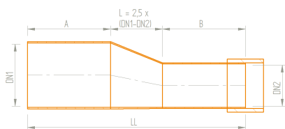
Redukcja ekscentryczna
