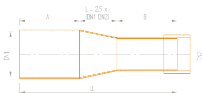
Redukcja koncentryczna
